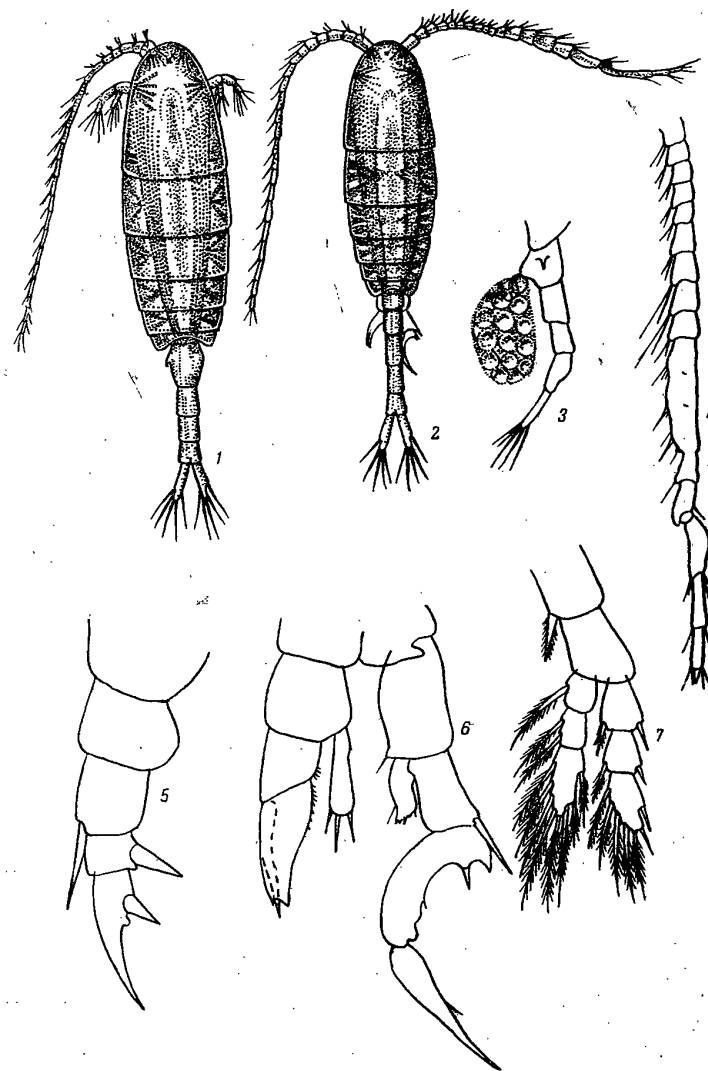
Рис. 179. Calanipeda aquae dulcis : 1 — общий вид самки; 2 — общий вид самца; 3 — abdomen самки, вид сбоку; 4 — геникулирующая антенна самки; 5 — V пара ног самки; 6 — V пара ног самца; 7 — IV пара ног самки (по G. O. Sars).
