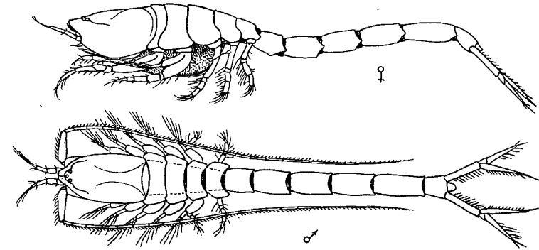
Рис. 251. Stenocuma gracilis (G. O. Sars).
