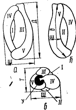
Рис. 35. Части квинквелокуляционной раковины и ее измерения: а — многокамерная сторона; б — малокамерная сторона; в — устьевая сторона; У — устье; Д — длина раковины; Т — толщина раковины; д — длина камеры; ш — ширина камеры; I, II, III, IV и V — камеры последнего наружного цикла (по А. Богдановичу, 1952, с изменением в нумерации камер наружного цикла).
