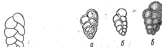
Рис. 38. Раковина с двухрядным расположением камер:
