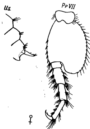
Рис. 279. Niphargoides (Pontogammarus) crassus (Grimm).
