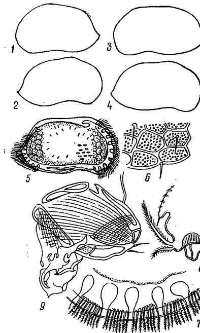
Рис. 212. Hemicythere sicula (Brady): 1 — очертание правой створки раковины самки; 2 — очертание левой створки раковины самки; 3 — очертание правой створки раковины самца; 4 — очертание левой створки раковины самца; 5 — правая створка раковины, вид сбоку; 6 — скульптура поверхности раковины; 7 — поровые каналы на переднем крае створки; 8 — фурка; 9 — копулятивный орган (1—5 по Бронштейну, 1947; 5—9 по Daday, 1904).
