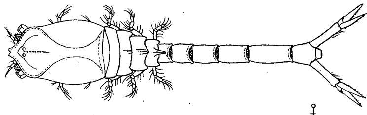
Рис. 242. Pterocuma grandis G. O. Sars.
