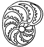
Рис. 29. Спиральноплоскостная полуэволютная раковина — Faujasinella .
