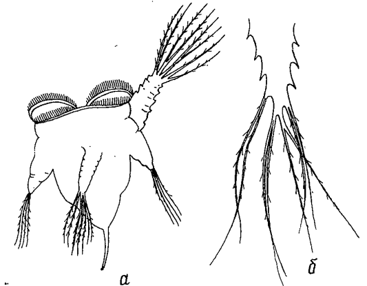
Рис. 116. Hexarthra oxyuris : а — общий вид (по Wiszniewski, 1932); б — брюшной вырост.
