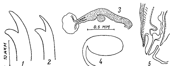
Рис. 131. Eulyodrilus caspicus Lastockin: 1 — брюшная щетинка V сегмента; 2 — спинная щетинка XXXI сегмента; 3 — семенная воронка, проксимальный конец атриума и простаты; 4 — семяприемник; 5 — проксимальные части мужских протоков (по Hgabei, 1950).
