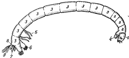
Рис. 328. Внешний вид личинки хирономид (род Chironomus ) (по Константинову, 1958): 1 — голова; 2 — грудные сегменты; 3 — брюшные сегменты; 4 — передние ложные ножки; 5 — мягкие выросты XI сегмента; 6 — задние ложные ножки; 7 — анальные папиллы; 8 — подставки кисточек; 9 — щетинка кисточек.
