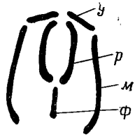
Рис. 91. Схема строения мастакса (по Donner, 1956): у — ункус; р — рамус; м — манубрий; ф — фулькрум.
