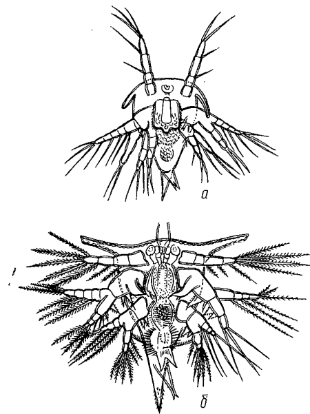
Рис. 188. Науплиусы Balanus improvisus : а — I стадия; б — II стадия × 360 (по Ноекс, 1909).
