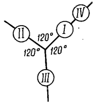
Рис. 33. Схема расположения камер клубкообразно-звернутых раковин трилокуляционного типа (по А. Богдановичу, 1952): I—IV — камеры.
