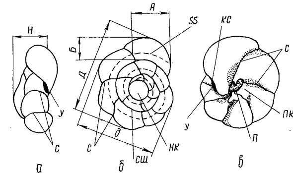
Рис. 32. Схема строения трохонидной спиральноконической раковины:
