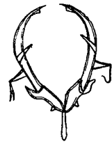
Рис. 114. Asplanchna brightwelli . Челюсти мастакса.
