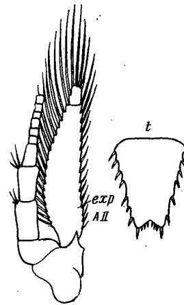
Рис. 235. Diamysis pusilla (G. O. Sars).
