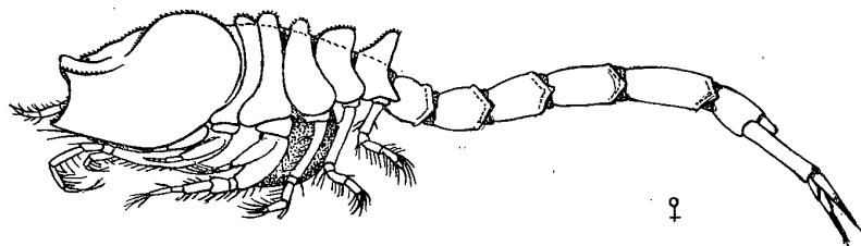
Рис. 243. Pterocuma rostrata (G. O. Sars).
