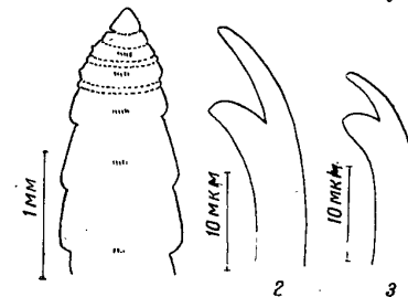
Рис. 133. Limnodrilus michaelseni Lastockin:
