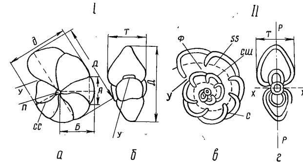
Рис. 28. Схема строения спиральноплоскостной инволютной раковины (по Н. А. Волошиновой, 1952, с некоторыми изменениями):
