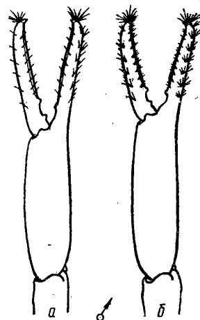
Рис. 323. Клешня ходильной ноги II пары пресноводных креветок Palaemon : а — P. adspersus ; б — P. elegans .
