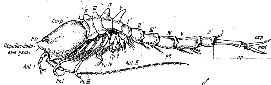
Рис. 237. Схема строения Pterocuma pectinata : Ant I ; Ant II — антенны; Pp I — Pp V — переоподы; Pl — плеоподы; ur — уropоды; t — тельсон; exp — экзоподит уropода; end — эндоподит уropода; Carp — карапакс; Psr — псевдорострум; I—V — свободные грудные сегменты; I'—VI' — сегменты брюшного отдела.
